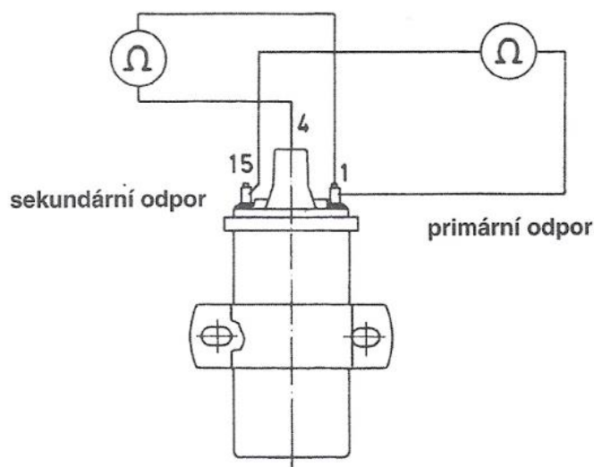
Obr. 6 Měření přerušení vinutí zapalovací cívky. [2]
